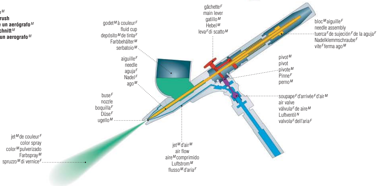
flexible M d'air M air hose conducto M de aire M comprimido Luftschlauch M tubo M flessibile per l'aria F
